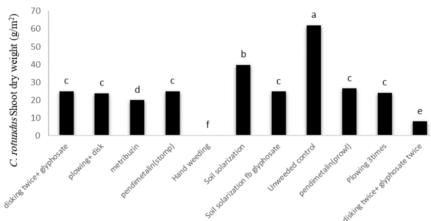
شکل ۳- اثر روش‌های مختلف مدیریت بر وزن خشک اندام هوایی اویارسلام ارغوانی
