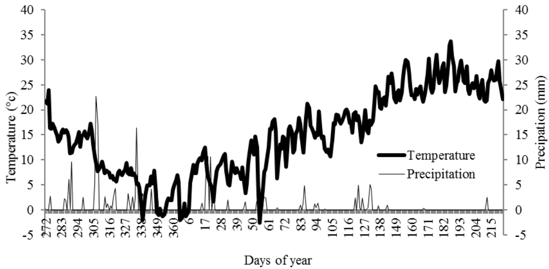
شکل ۱- میزان بارندگی و دمای کمینه و بیشینه در عمق ۵ سانتی متری خاک در طول فصل زراعی ۱۳۹۱-۱۳۹۲
